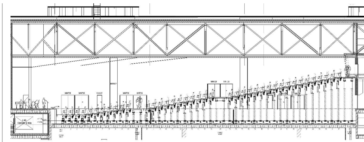
Metszeti rajz:
