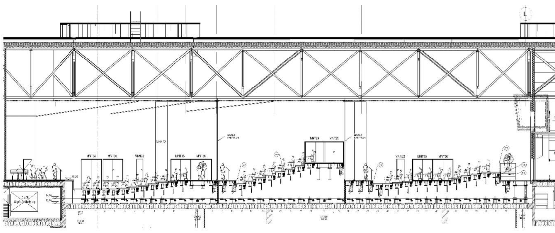
Metszeti rajz:
